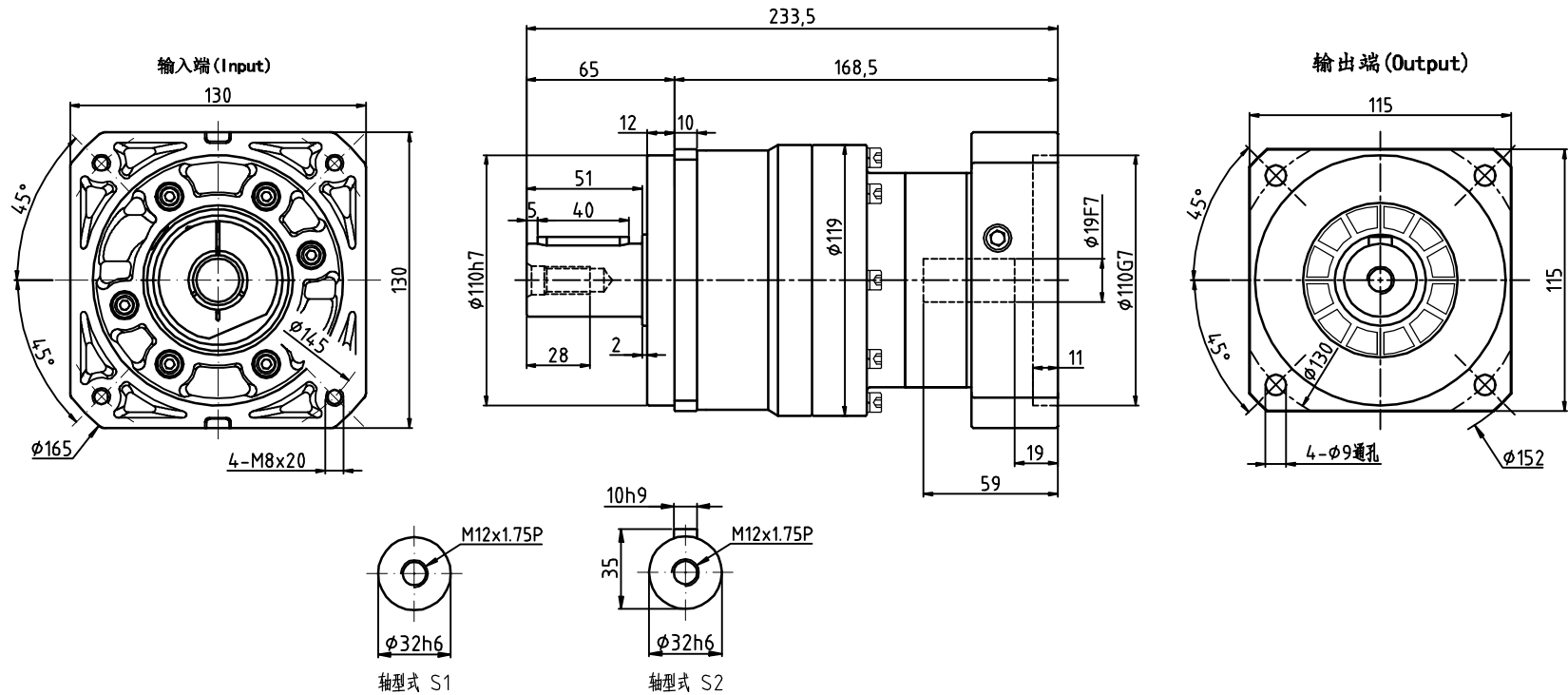
尺寸图
